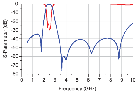
RFBPF2012040ABT
